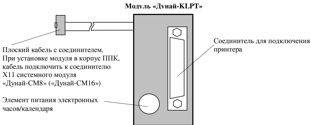
Рисунок Г.5 – Подключение внешних цепей к модулю «Дунай-КЛРТ»
