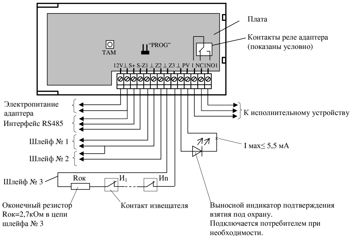
Рисунок Г.10 – Пример подключения адаптера «Дунай-АД3»
