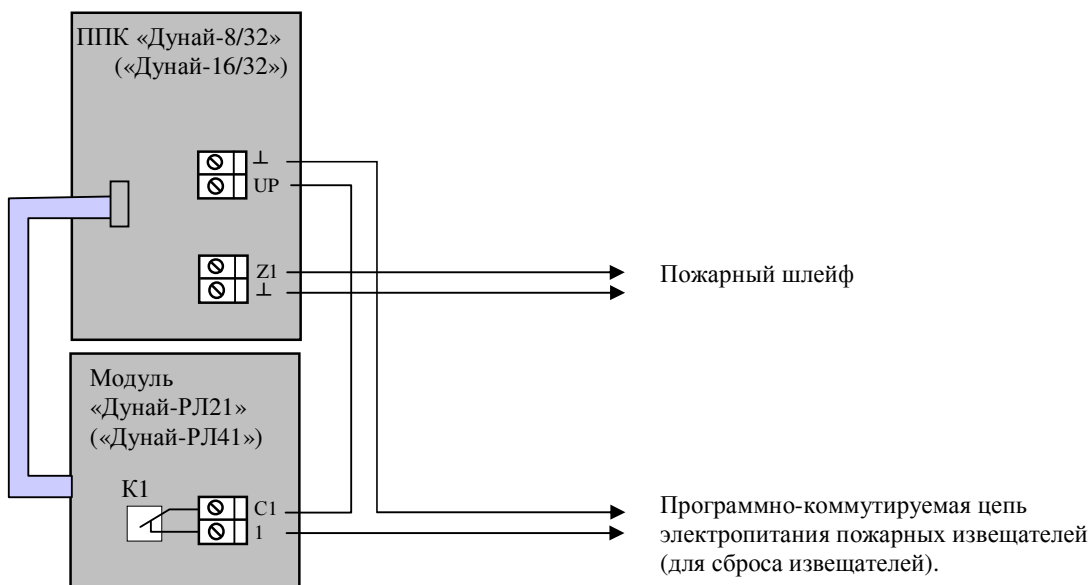
Рисунок Е.4 – Схема организации программно-коммутируемой цепи электропитания пожарных извещателей при использовании модулей «Дунай РЛ21» («Дунай РЛ41»)
