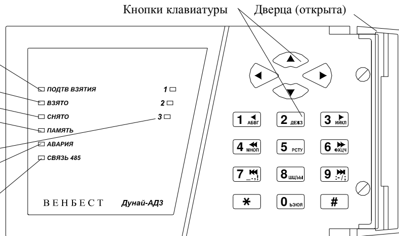
Рисунок Б.6 – Схема размещения кнопок и индикаторов в адаптере «Дунай-АДЗ»
