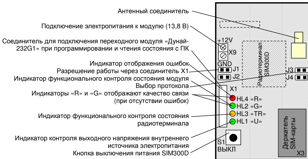
Рисунок В.4 – Вид модуля «Дунай-G2»
