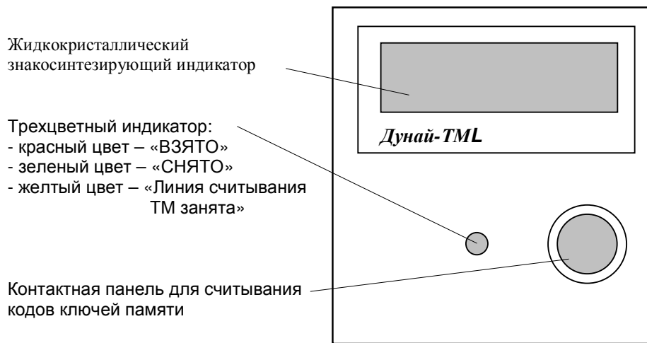
Рисунок Б.7 – Вид адаптера «Дунай-TML»
