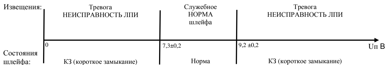
Рисунок Д.2 – Структура шлейфа контроля ЛПИ
