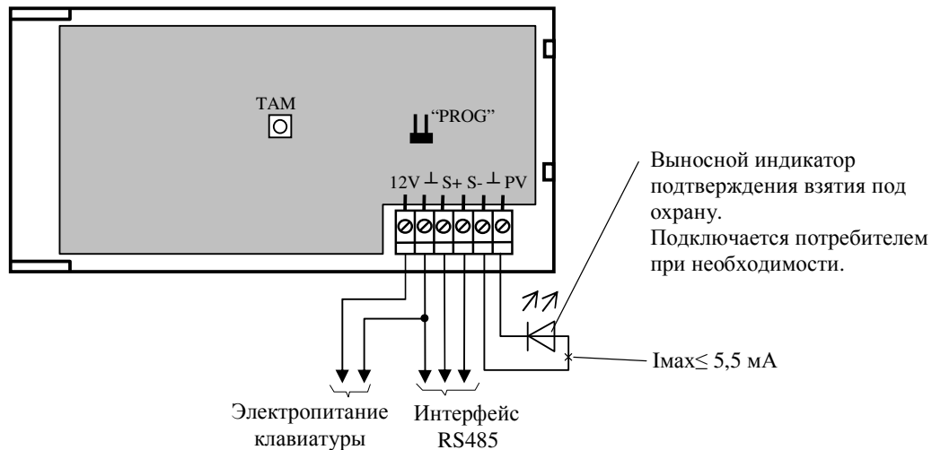
Рисунок Г.9 – Пример подключения клавиатур «Дунай-КС8», «Дунай-КС16», «Дунай-КЖ»
