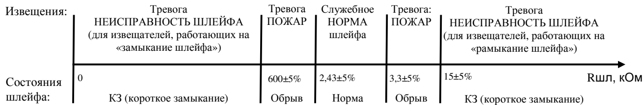
Рисунок Д.1 – Структура активного пожарного шлейфа
