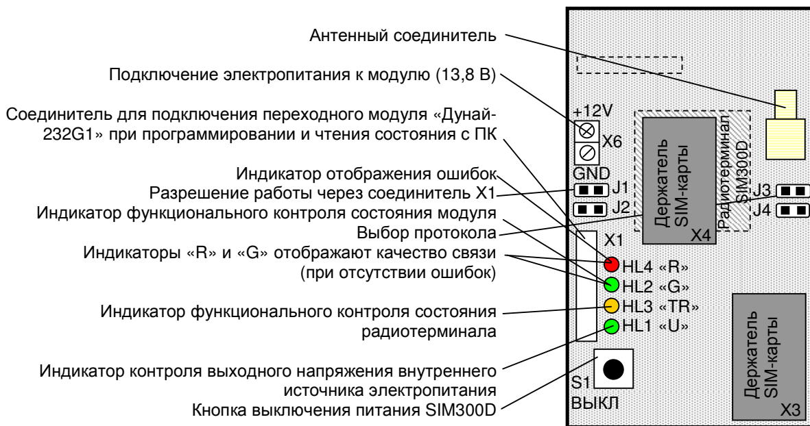
Рисунок В.5 – Вид модуля «Дунай-G2S»
