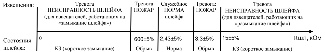
Рисунок Д.1 – Диаграмма формирования извещений при изменении сопротивления пожарного шлейфа
