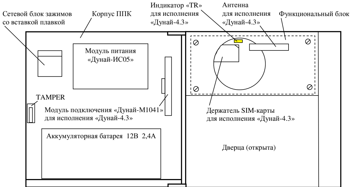
Рисунок Б.1 – Размещение модулей в ППК
