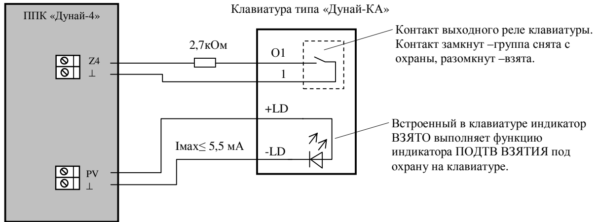
Рисунок Ж.1 – Пример подключения к ППК клавиатуры с выходным реле
