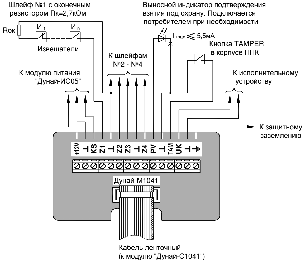
Рисунок Г.3 – Вид модуля «Дунай-М1041» для исполнения «Дунай-4.3»
