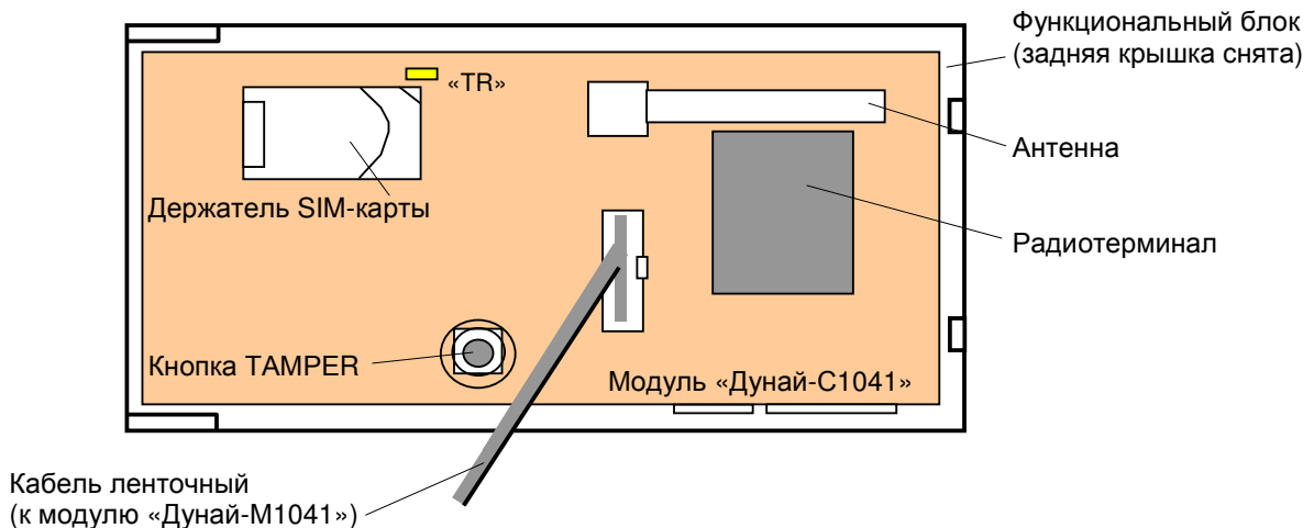
Рисунок Г.2 – Вид модуля «Дунай-С1041» для ППК исполнения «Дунай-4.3»
