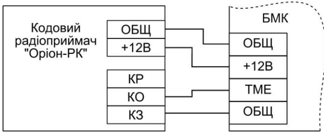
Рисунок 4 - Схема підключення кодового радіоприймача «Оріон-РК»
