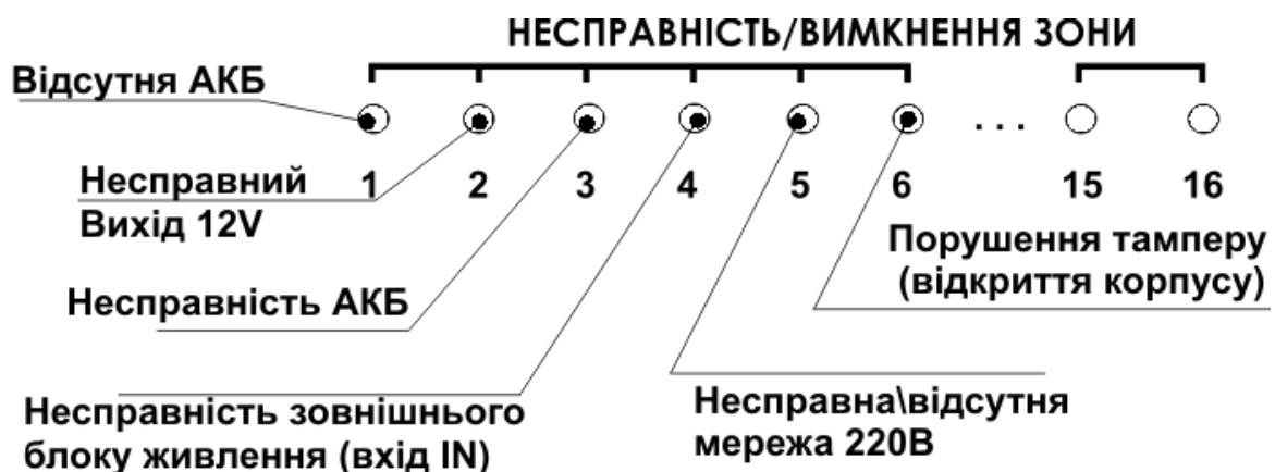
Рисунок 5.2 – Розширена індикація несправностей живлення
